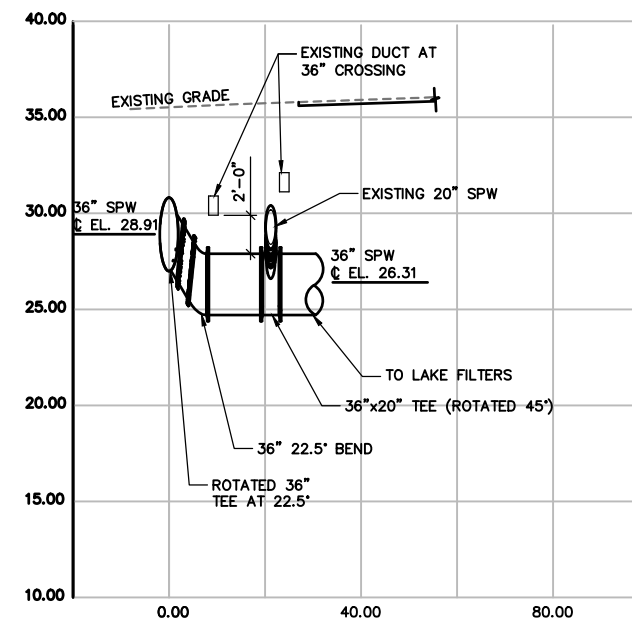
PROFILE-B SCALE: 1" = 20' HORIZ. 1" = 5' VERT.
