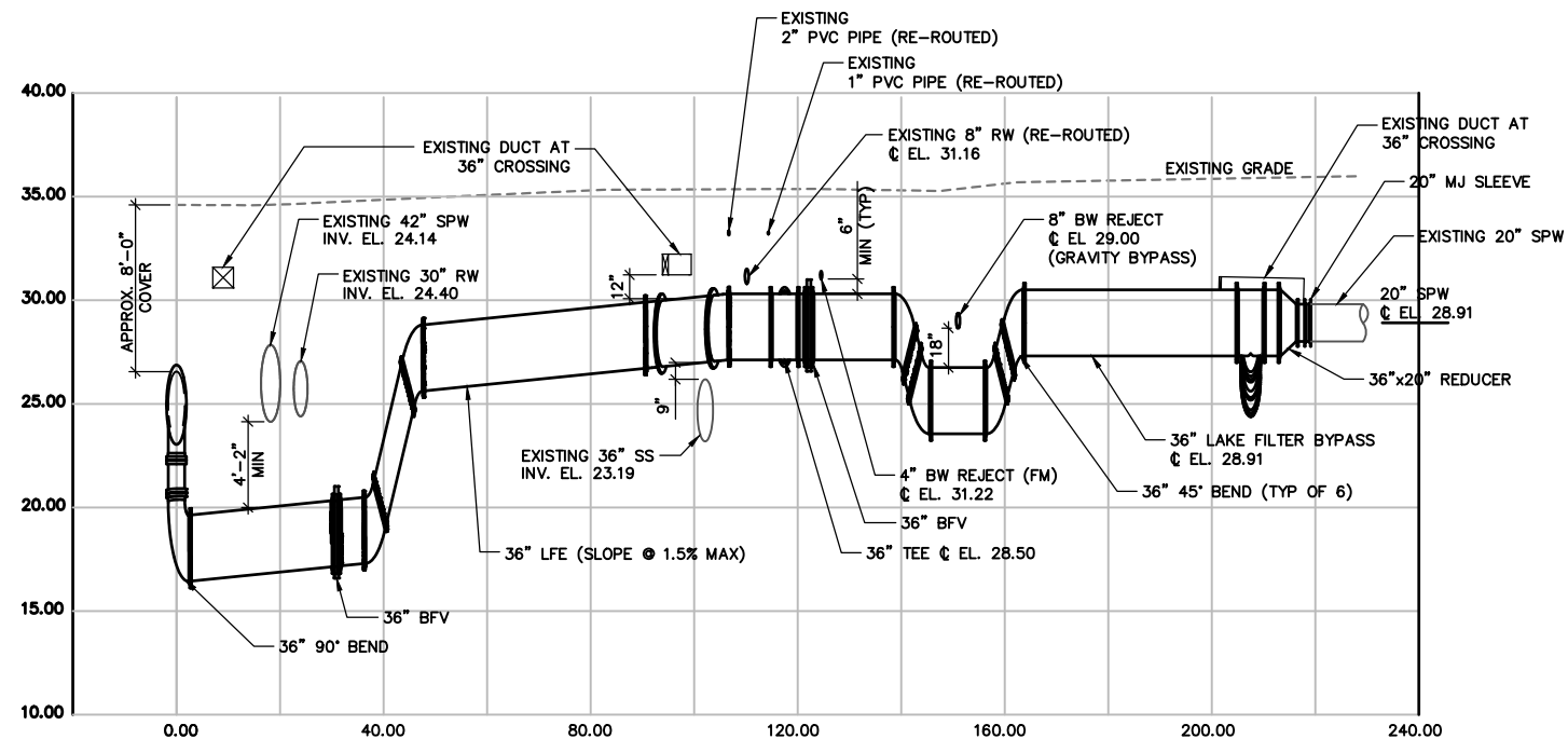
PROFILE-A SCALE: 1" = 20' HORIZ. 1" = 5' VERT.
